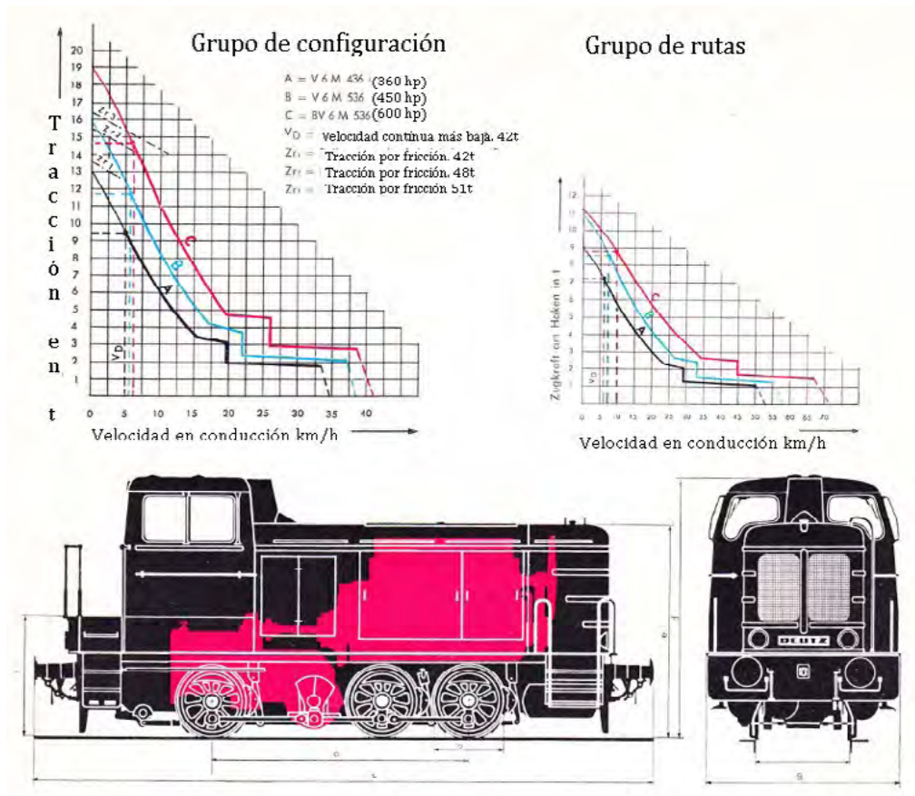
Locomotora de tracción diesel-hidráulica VW-62
